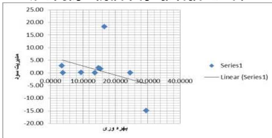
نمودار ۱۹ نتیجه آزمون رگرسیون خطی و نمودار توزیع پراکندگی برای فرضیه دوم
